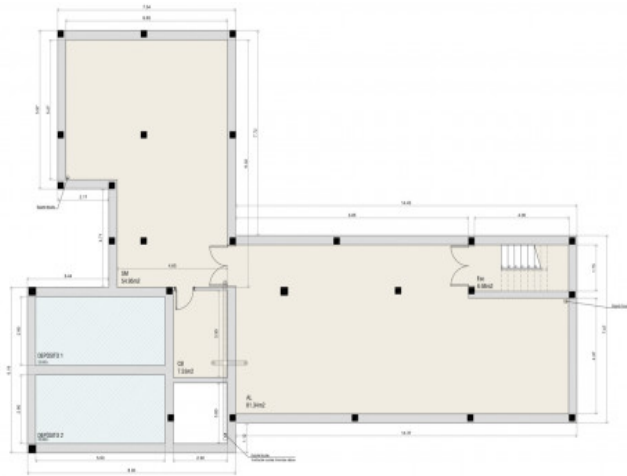
SUPERFICIE CONSTRUIDA DE GOTANCO=710M2 PLANTA GOTANCO E: 1/50
